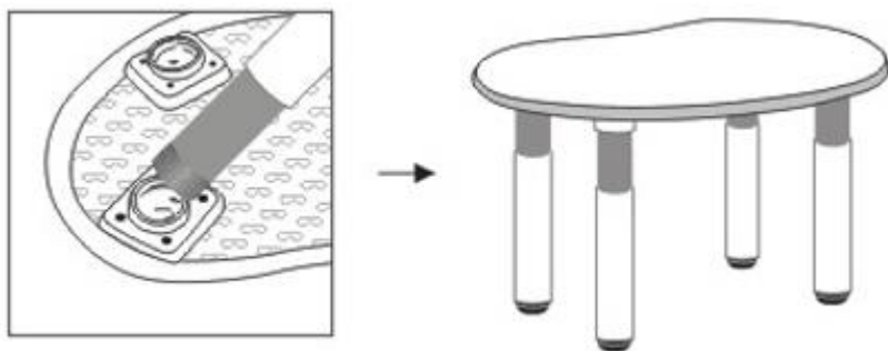
Upevnenie nôh do dosky stola.
